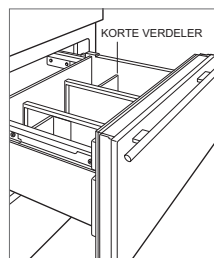
Ladeschotten
