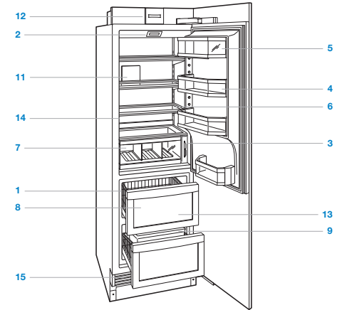
Combinazione a colonna.
