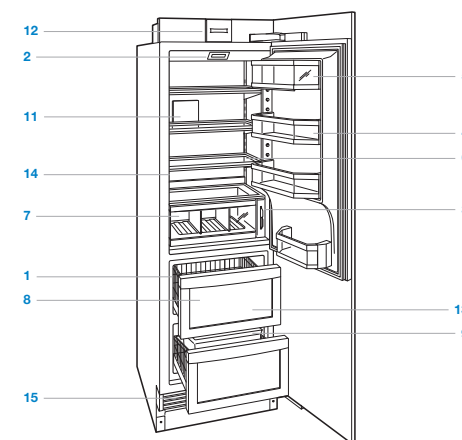
Modèle en colonne combiné
