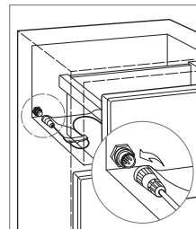
Steuerkabel (Schubladen)
