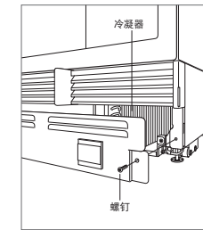
冷凝器位置。
