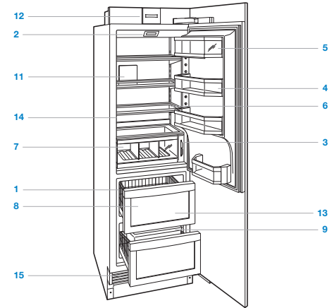
Combinación de la columna.
