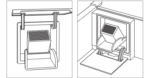
Cartucho del sistema de purificación de aire (alto y de columna).
