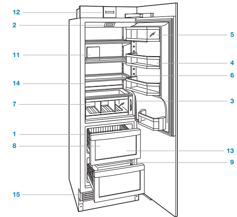
Säulenkombinationsmodell
