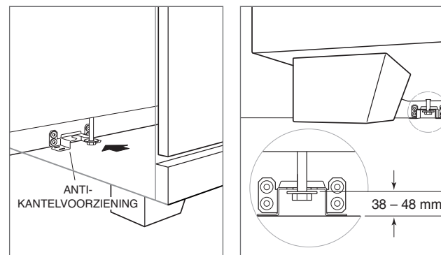
Locatie anti-kantelvoorziening
