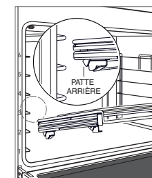
Installez la grille multifonctions
