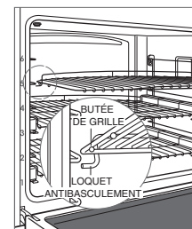
Dispositif antibasculement de la grille du four
