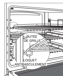
Dispositif antibasculement de la grille du four
