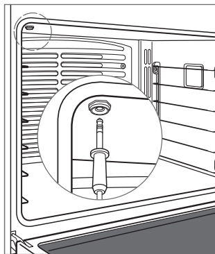
Probe receptacle
