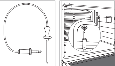
Sensor de temperatura Receptáculo para sensor de temperatura
