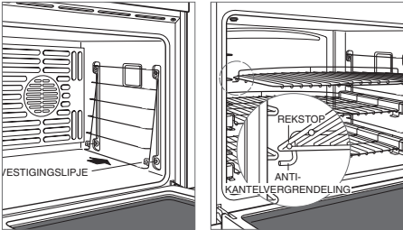
Ovenrekgeleider
