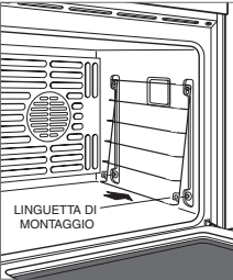
Guida della griglia del forno
