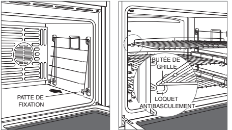
Guide-grilles du four Dispositif antibasculement de la grille du four
