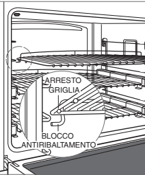
Blocco antiribaltamento della griglia del forno
