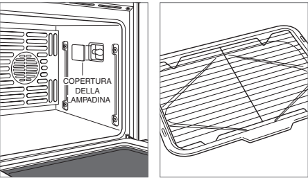
Sostituzione della lampadina Vaschetta della graticola e griglia
