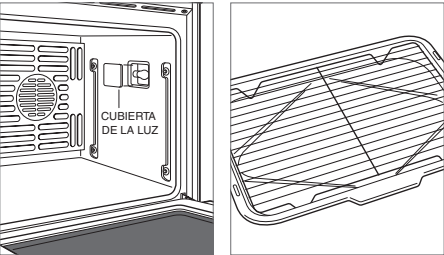
Cambio de la bombilla Bandeja para asar y rejilla
