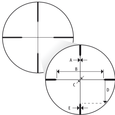
Präzisionsfadenkreuz
