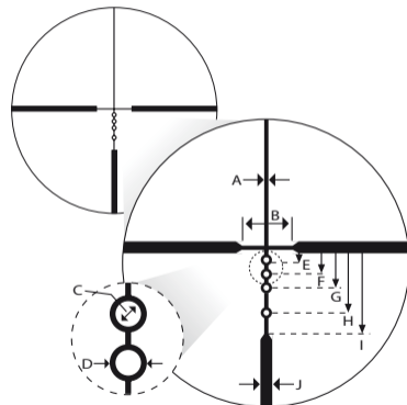
Réticule BDC 150
