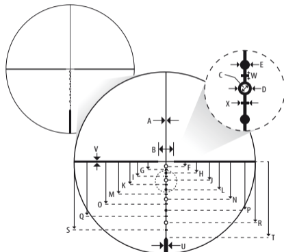
Réticule BDC 800
