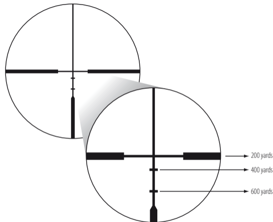
Réticule BDC Carbine
