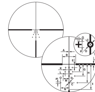
Rozšířený záměrný kříž BDC
