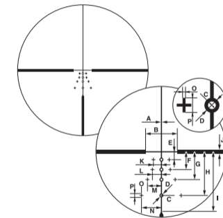
Retícula BDC avanzada
