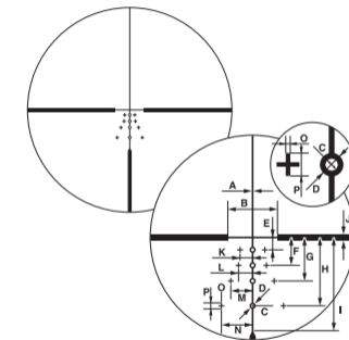
Kompaktes BDC-Fadenkreuz
