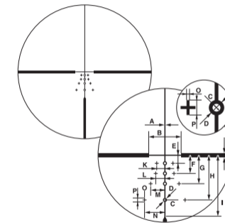
Retículo BDC avançado
