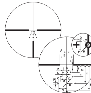
Zaawansowana siatka celownicza BDC
