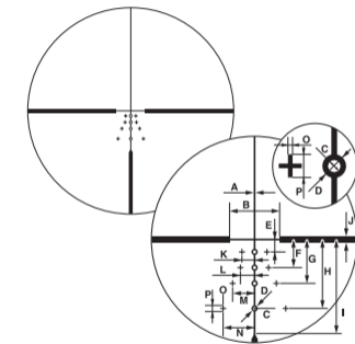
Réticule BDC perfectionné
