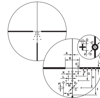
Avanceret BDC-trådkors
