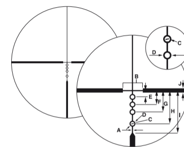
Réticule BDC standard
