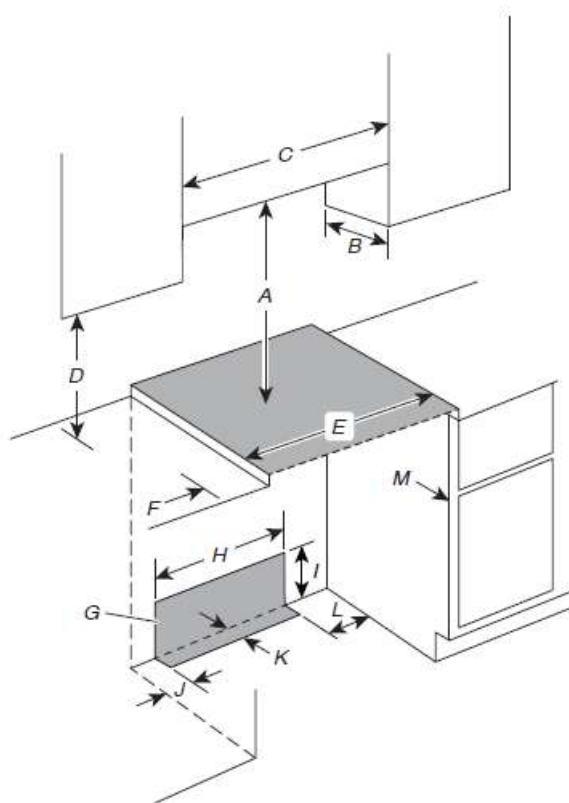
Ouverture pour les commandes frontales
