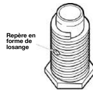
Pied de nivellement avec repère en forme de losange
