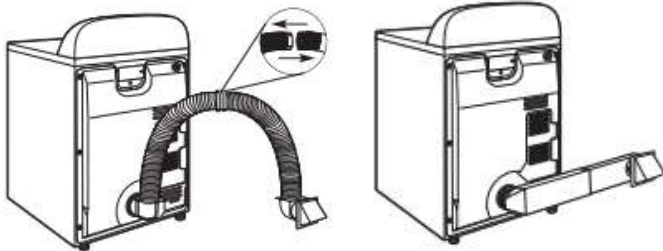
Installation au-dessus de la sèche-linge (également offerte avec un coude décalé) Installation en périscopie
