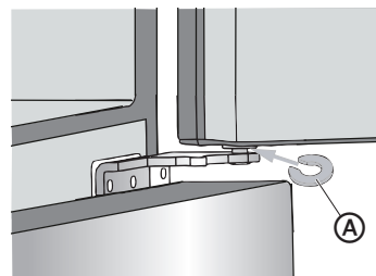
Ⓐ Entretoise (fournie)
