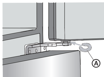
Ⓐ Espaciador (provisto)
